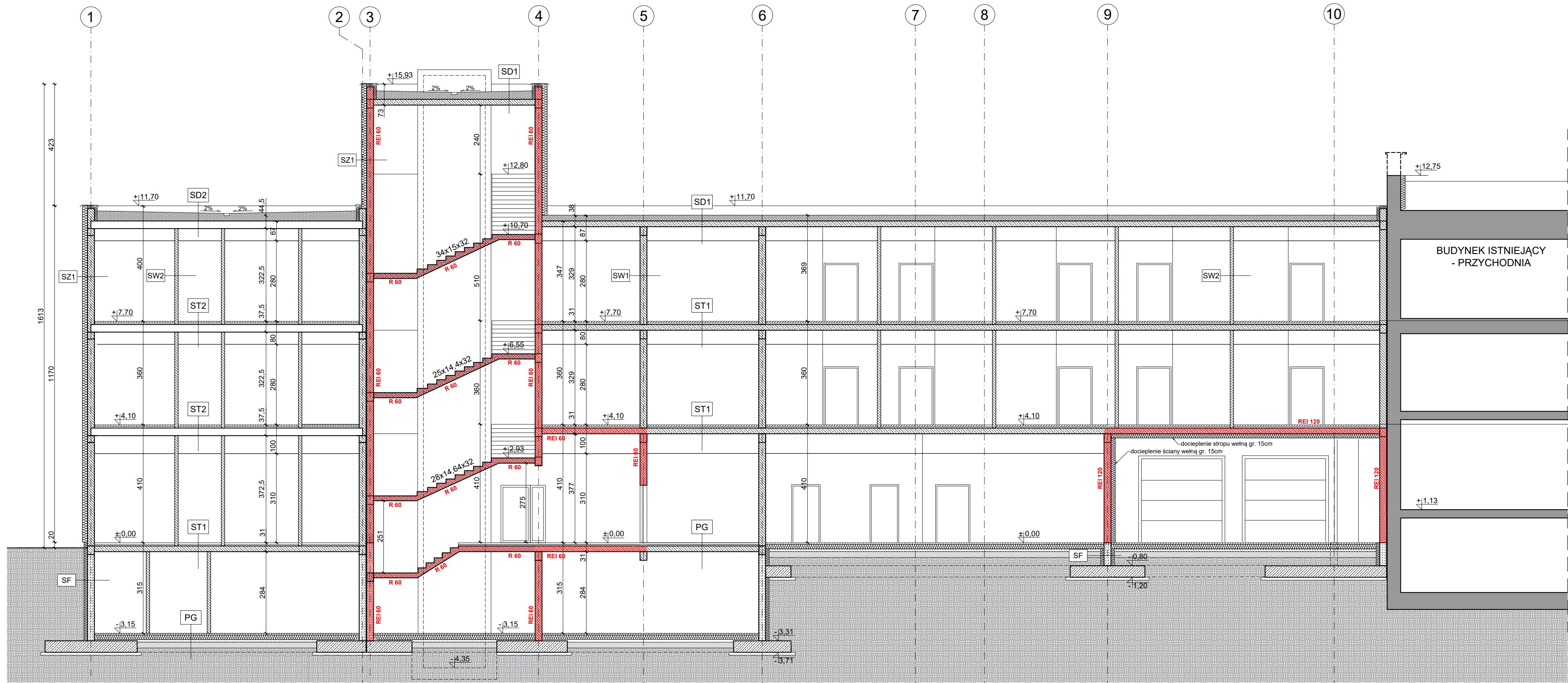
PRZEKRÓJ A-A
